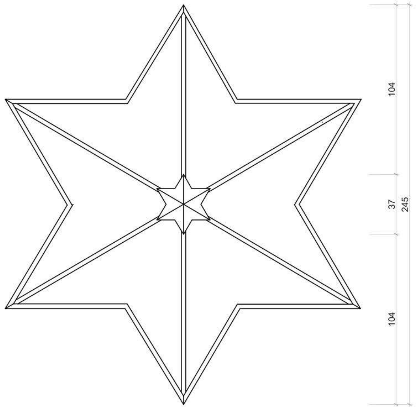
Rzut, 1:20
