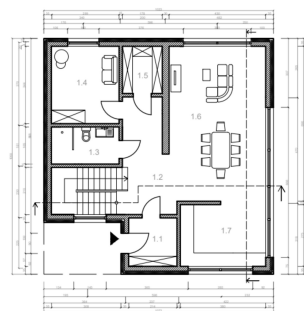
Rzut parteru, 1:100
