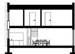
Przekrój B-B, 1:100
