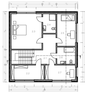
Rzut piętra, 1:100
