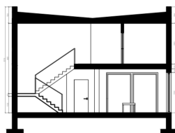
Przekrój A-A, 1:100
